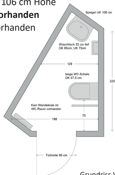
Grundriss WC
