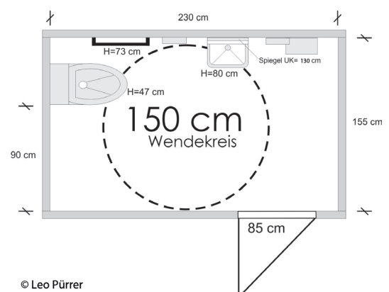
WC Plan
