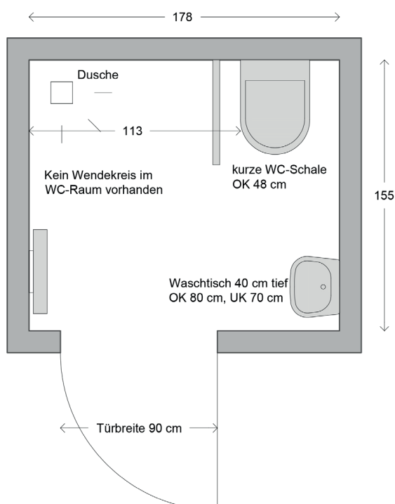
Grundriss WC
